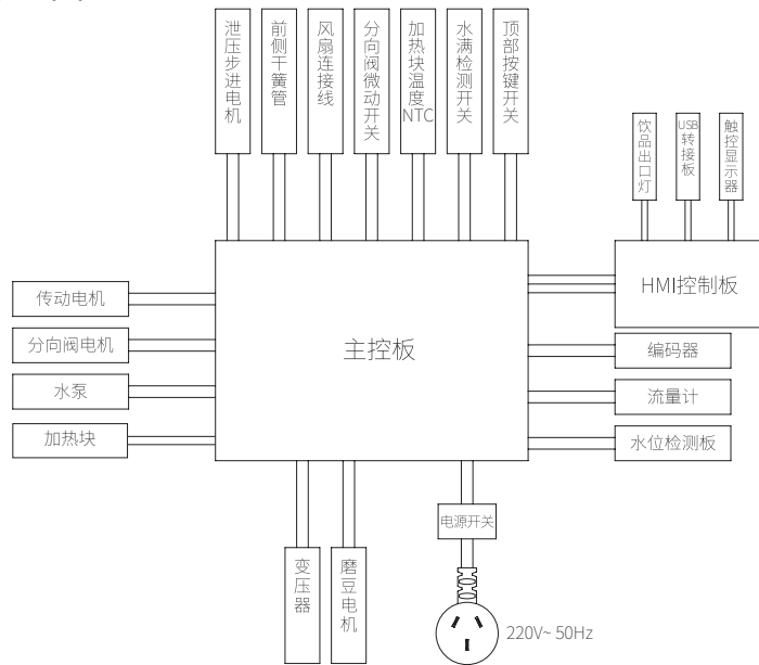
电气原理图
